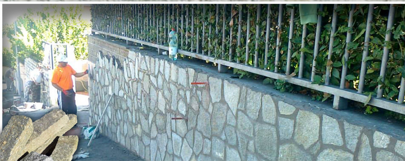
PIETRA DI LUSERNA - OPERA INCERTA
