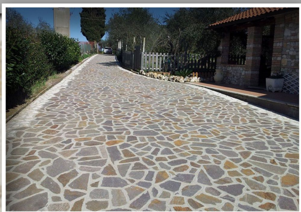
LASTRE DI PORFIDO OPERA INCERTA CON GRECA IN TRANI
